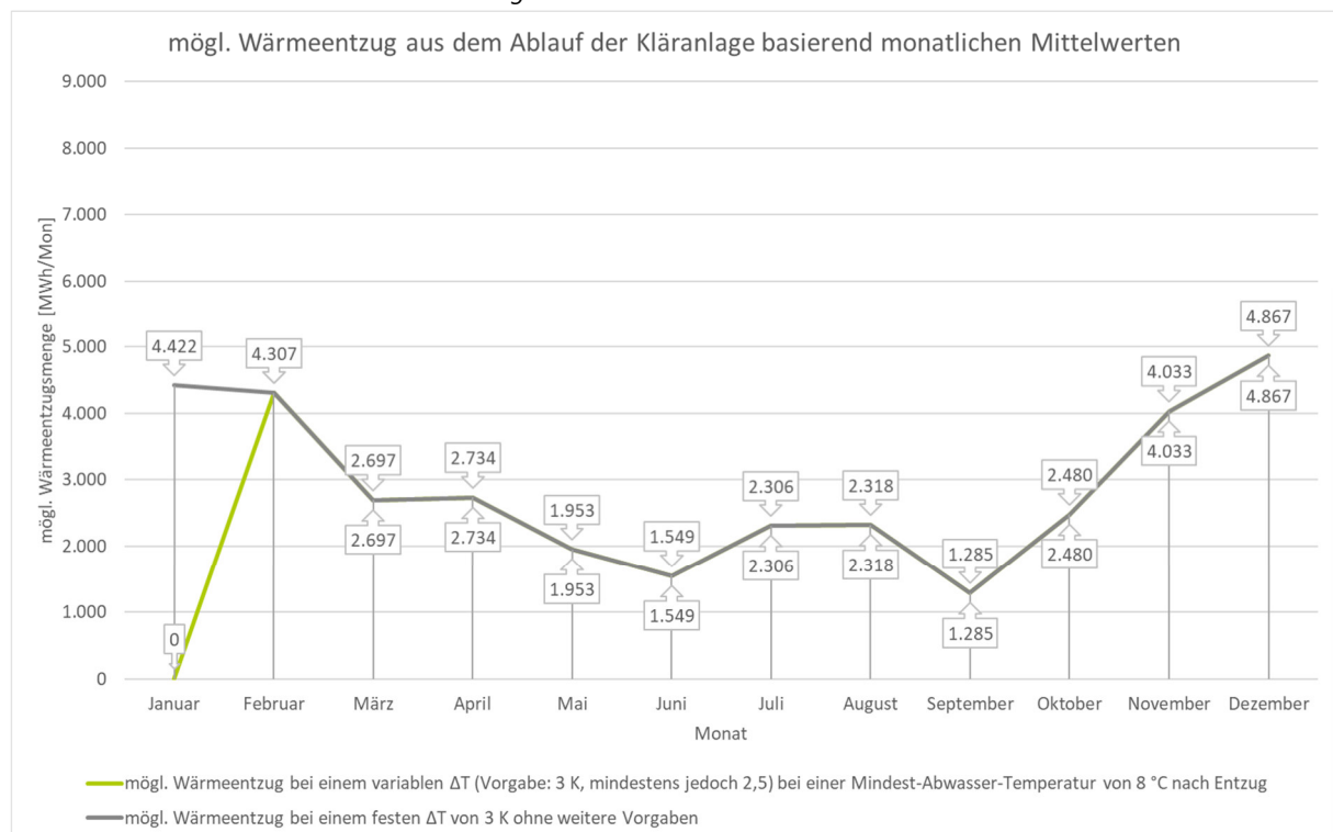
Anhang 18: Möglicher rechnerischer Wärmeentzug für gemittelte Werte 2023/2024 mit monatlichen Mittelwerten Szenario 6 - Diagramm
