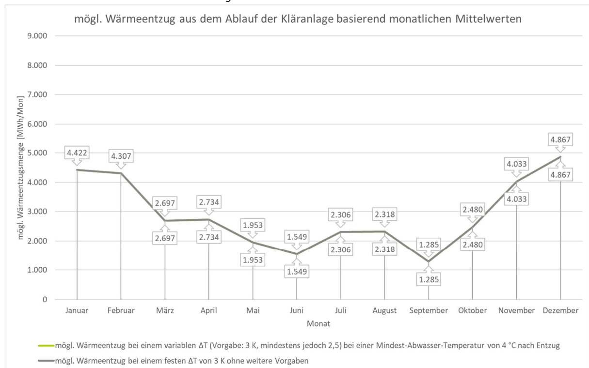
Anhang 14: Möglicher rechnerischer Wärmeentzug für gemittelte Werte 2023/2024 mit monatlichen Mittelwerten Szenario 4 - Diagramm
