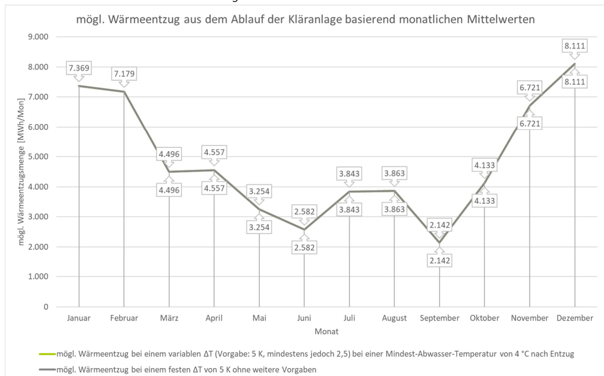
Anhang 8: Möglicher rechnerischer Wärmeentzug für gemittelte Werte 2023/2024 mit monatlichen Mittelwerten Szenario 1 – Diagramm
