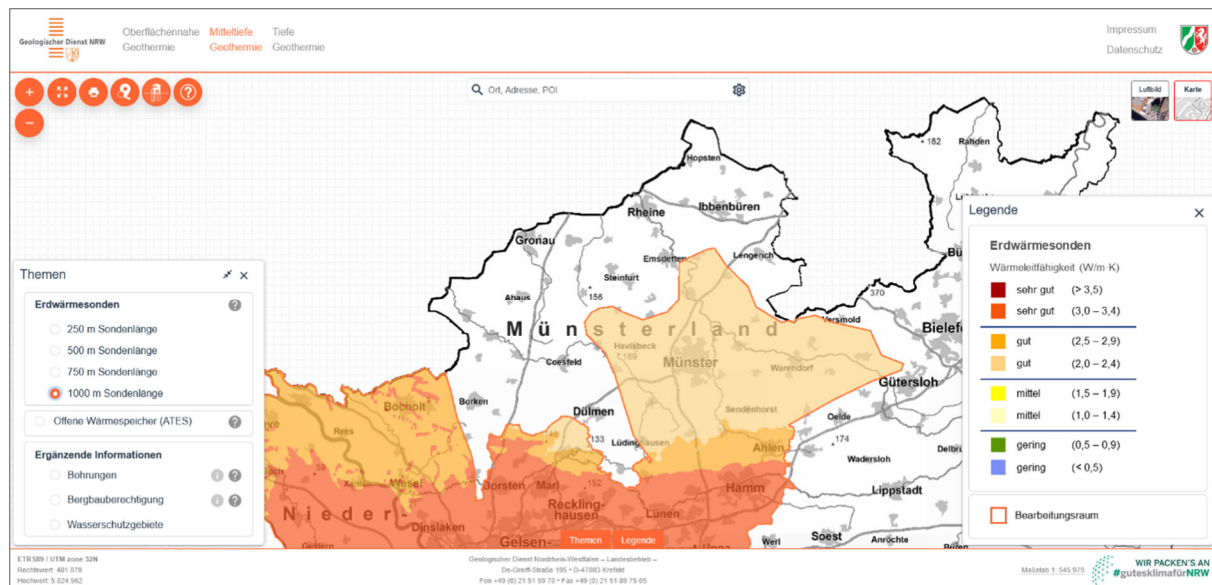
Abbildung IV-42: Wärmeleitfähigkeit (in W/(m·K)) des Untergrundes in NRW für Erdwärmesonden mit einer Sondenlänge von 1.000 m. Gronau liegt nicht im erfassten Gebiet. Quelle: Geologischer Dienst NRW.
