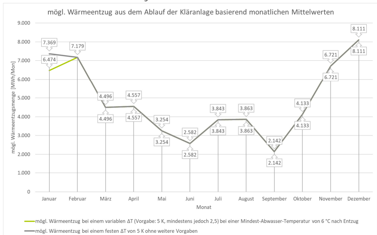
Anhang 10: Möglicher rechnerischer Wärmeentzug für gemittelte Werte 2023/2024 mit monatlichen Mittelwerten Szenario 2 - Diagramm
