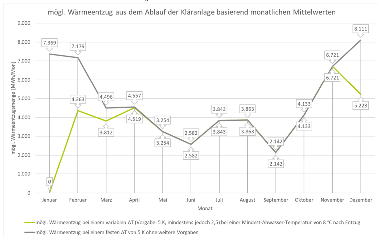
Anhang 12: Möglicher rechnerischer Wärmeentzug für gemittelte Werte 2023/2024 mit monatlichen Mittelwerten Szenario 3 - Diagramm
