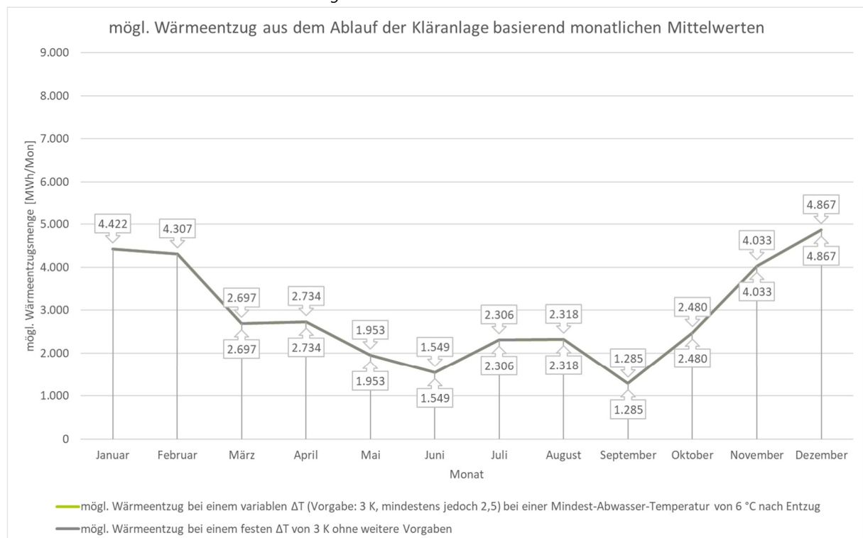
Anhang 16: Möglicher rechnerischer Wärmeentzug für gemittelte Werte 2023/2024 mit monatlichen Mittelwerten Szenario 5 - Diagramm
