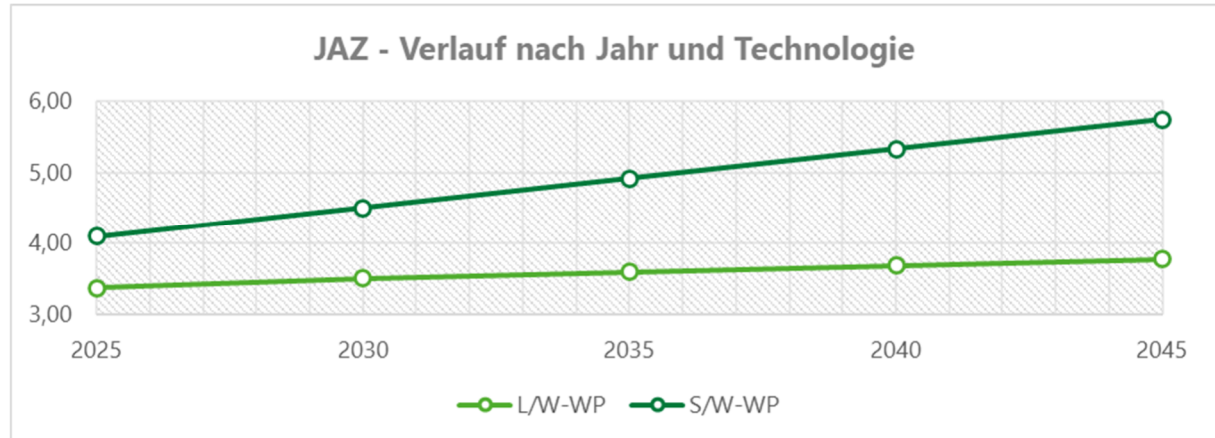
Abbildung V-6: angesetzte Entwicklung der Jahresarbeitszahl (JAZ) für Luft-Wasser-Wärmepumpen (L/W-WP) und Sole-Wasser-Wärmepumpen (S/W-WP; für Geothermie) über die Stützjahre zum Zieljahr anhand der Angaben des Technikkatalogs der KWW Halle.
