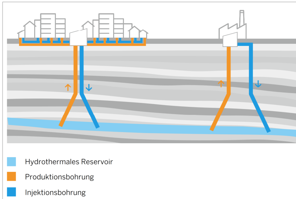
Abbildung IV-44: Tiefe Geothermie mittels hydrothormaler Dublette. Quelle: MWIKE NRW
