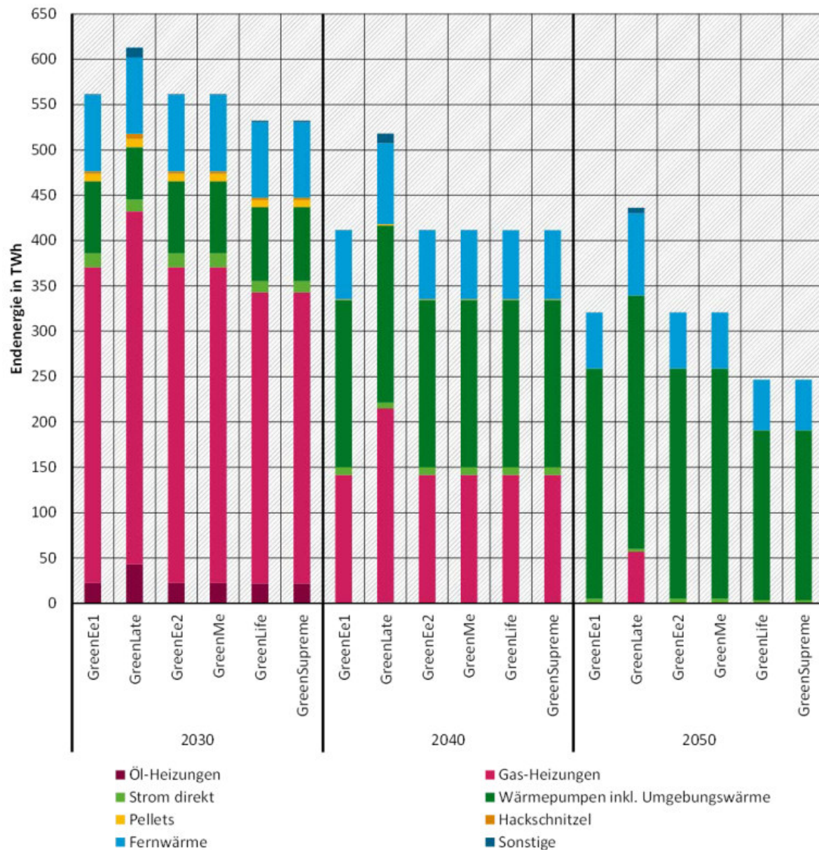
Abbildung V-4: Entwicklung der Endenergie nach Heiztechniken in den verschiedenen Green-Szenarien. Quelle: RESCUE – Studie (UBA)
