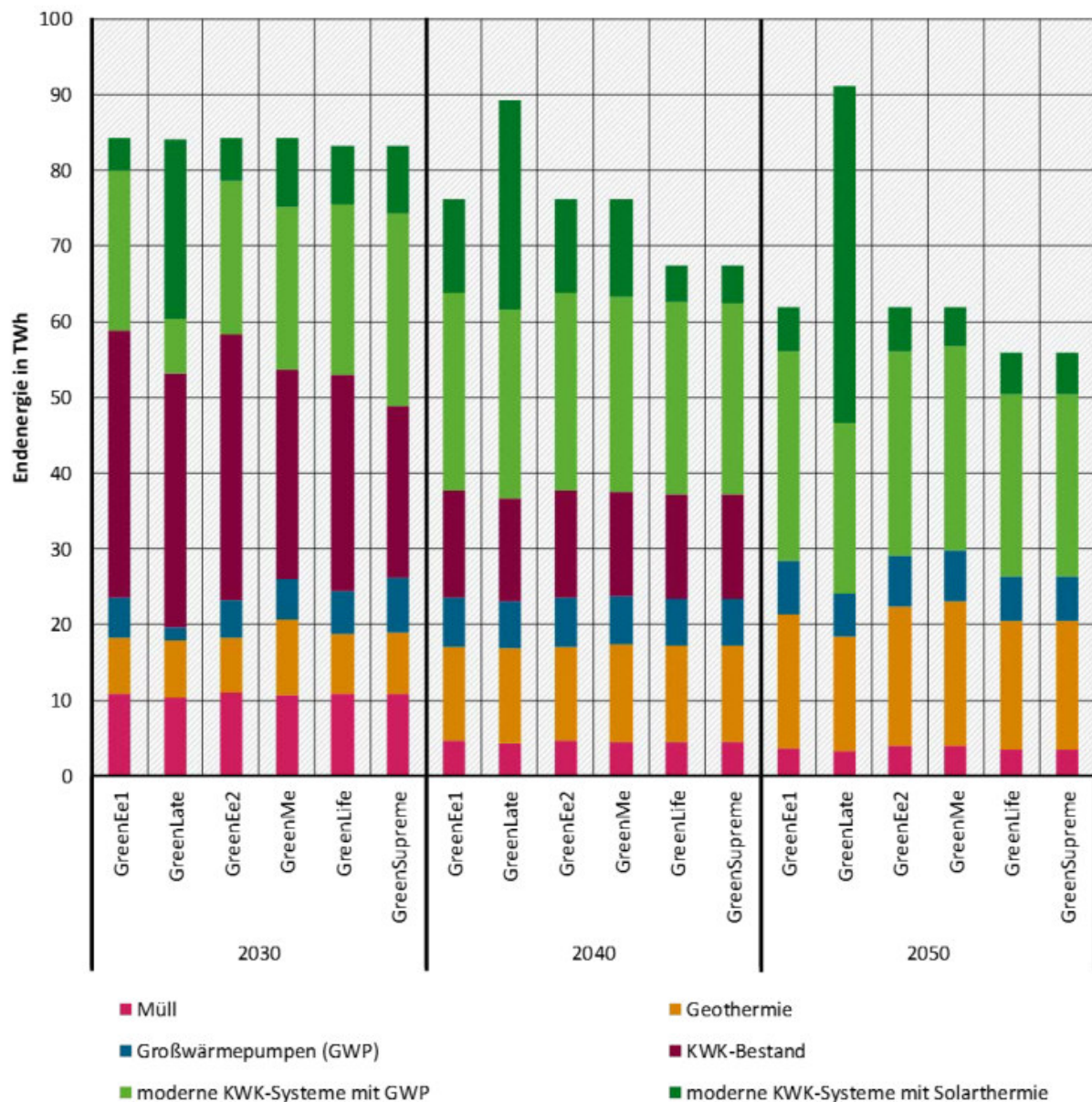
Abbildung V-5: Entwicklung der leitungsgebundenen Wärmeversorgung in den verschiedenen Green-Szenarien. Quelle: RESCUE – Studie (UBA)
