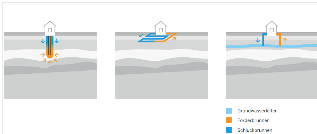
Abbildung IV-33: Oberflächennahe Geothermie mittels Erdwärmesonde (links), Erdwärmekollektor (Mitte), Brunnensystem (rechts). Quelle: MWIKE NRW
